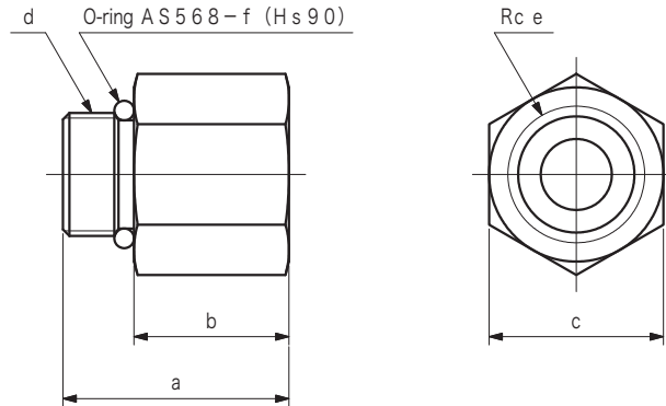
Dimensions table
